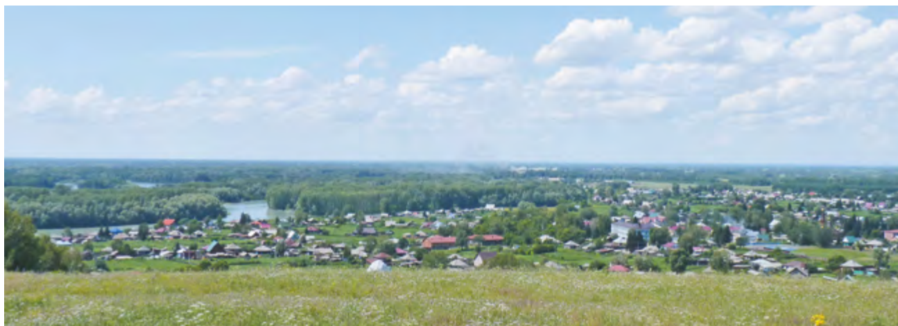
Вид с горы Пикет на Катунь, с. Сrostки
